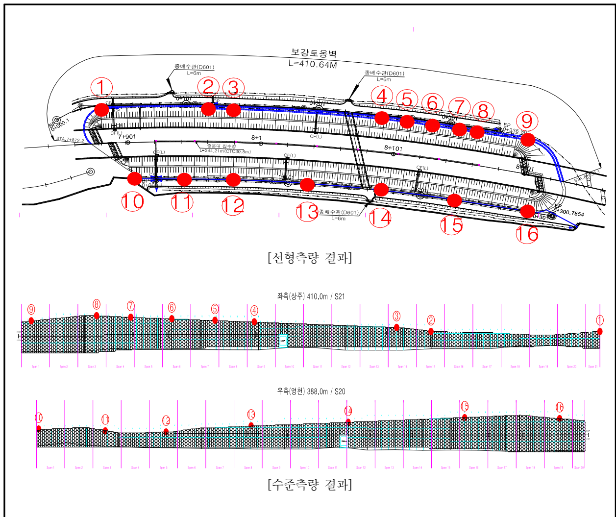
【그림 12.3.5】 선형 및 수준측량 결과
